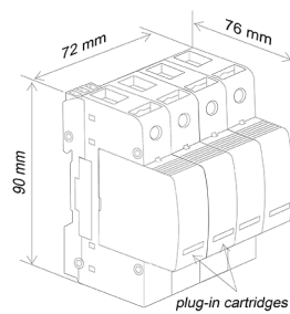
Zweipolig
