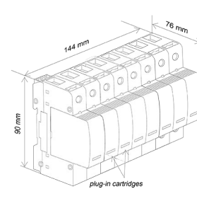
Vierpolig
