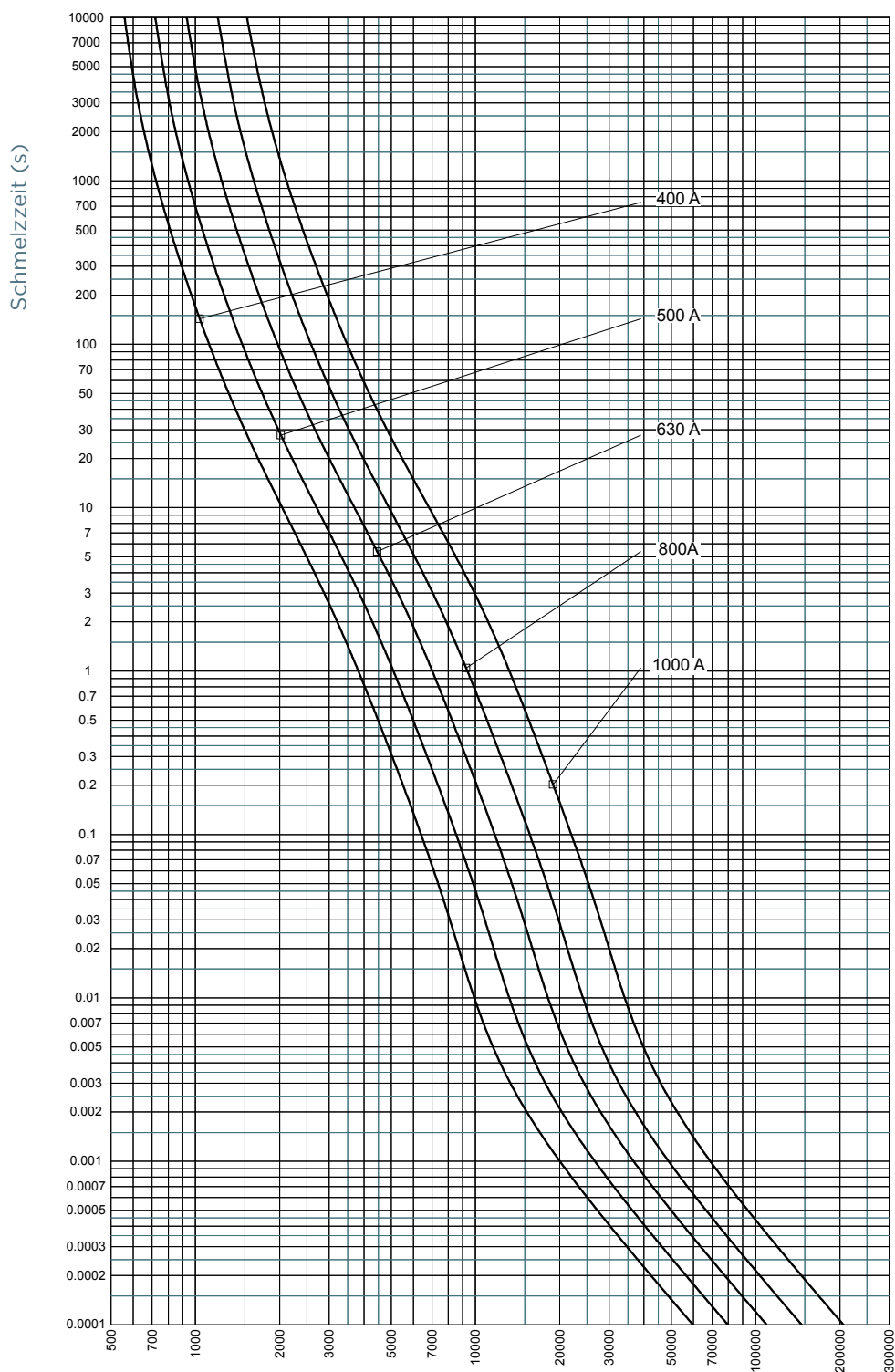
Effektivwert des Schmelzstroms (A) +/- 8%
