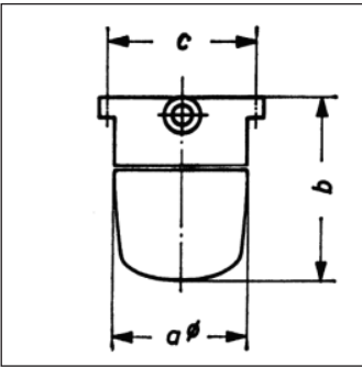
UNIFIX-Deckenleuchte
