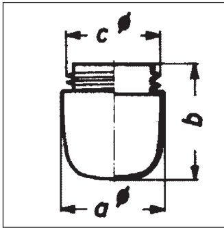
LISILUX-Ersatzschraubglas
