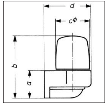
Saunaleuchte 6061
