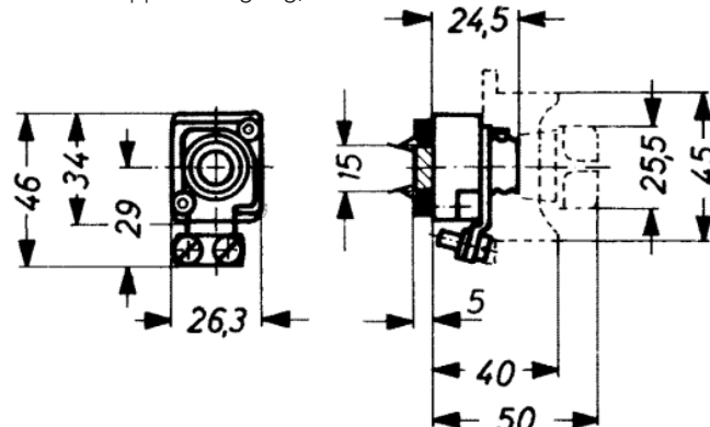
NEOZED-Reiter-Sicherungssockel mit Schnappbefestigung, ~400V
