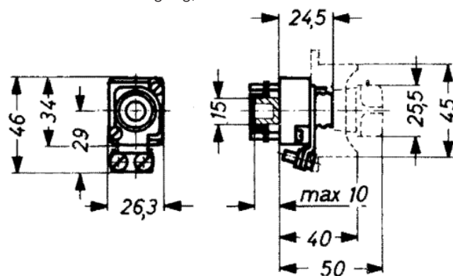
NEOZED-Reiter-Sicherungssockel mit Schellenbefestigung, ~400V
