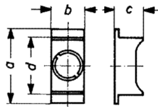
NEOZED Abdeckungen
