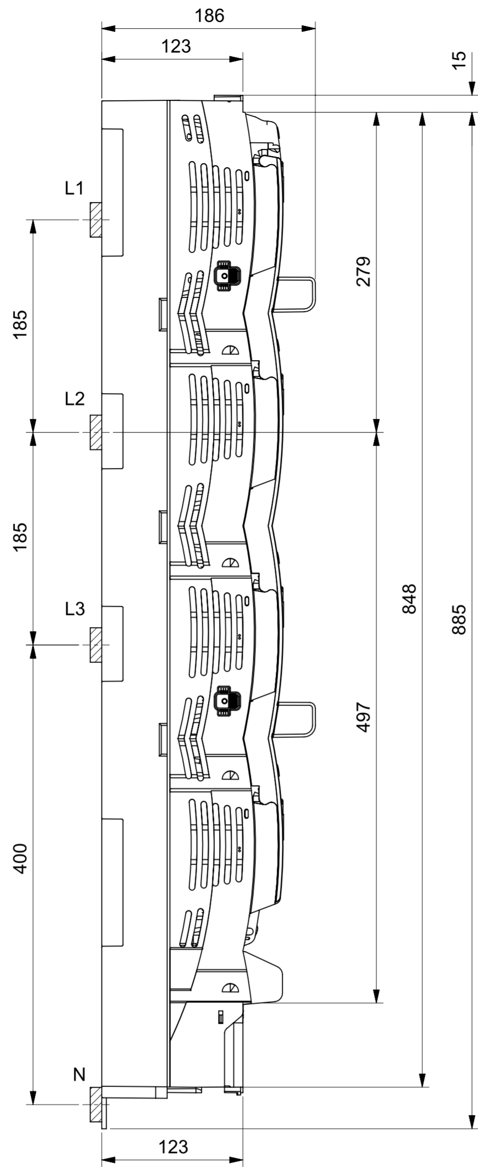
Variante mit erhöhter Abdeckklappe für die Nachrüstung von V-Anschlussbügeln
