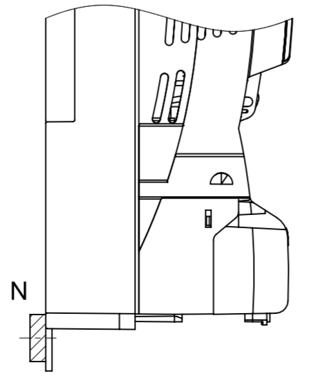
Variante mit erhöhter Abdeckklappe für die Nachrüstung von V-Anschlussbügeln
